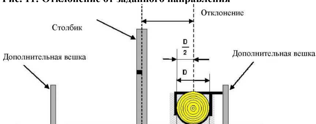
Рис. 11: Отклонение от заданного направления
