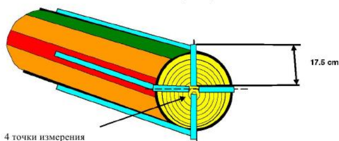
Рис. 23: Измерение углов и длина линейки
