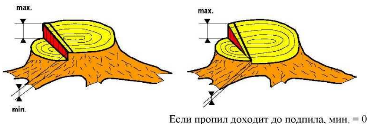
Рис. 15: Высота (минимум = 0 мм)
